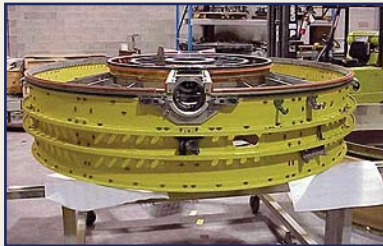
Fan Case
